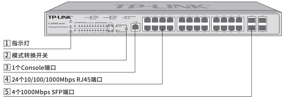
图1-12 TL-NS650-24GP4F前面板示意图
