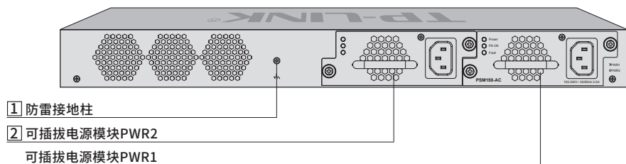
图1-13 TL-NS680-24T2Q后面板示意图
